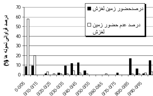
شکل ۳. درصد فراوانی حضور و عدم حضور لغزش در طبقات احتمال مختلف
