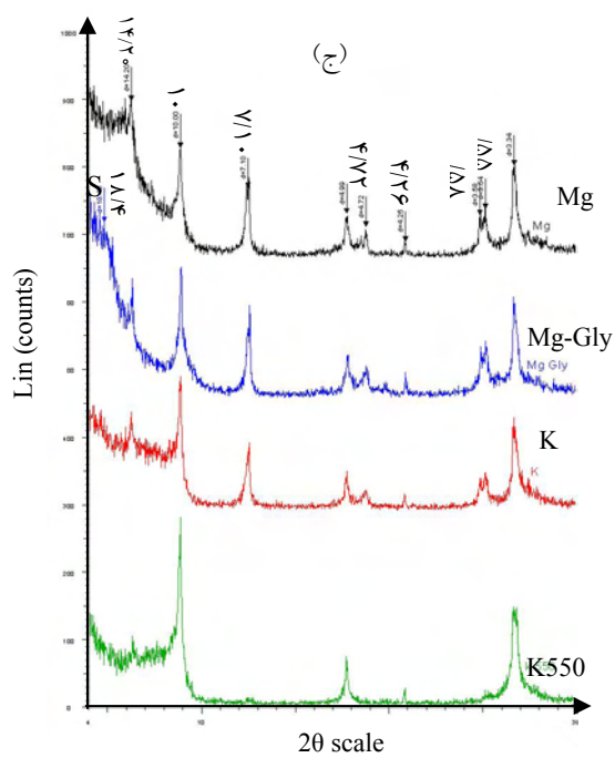
شکل ۳. نمونه‌هایی از تفرق اشعه ایکس الف: افق By پروفیل ۱، ب: افق Byz پروفیل ۲، ج: افق Byg 1 پروفیل ۳، که در تیمار منیزیم گلیسرول ظهور پیک ۱۸/۴ نشانه‌ای بر وجود اسمکتیت است.
