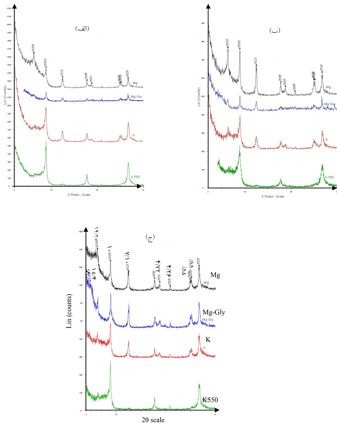
شکل ۳. نمونه‌هایی از تفرق اشعه ایکس الف: افق By پروفیل ۱، ب: افق Byz پروفیل ۲، ج: افق Byz 1 پروفیل ۳، که در تیمار منیزیم گلیسرول ظهور پیک ۱۸/۴ نشانه‌ای بر وجود اسمکتیت است.
