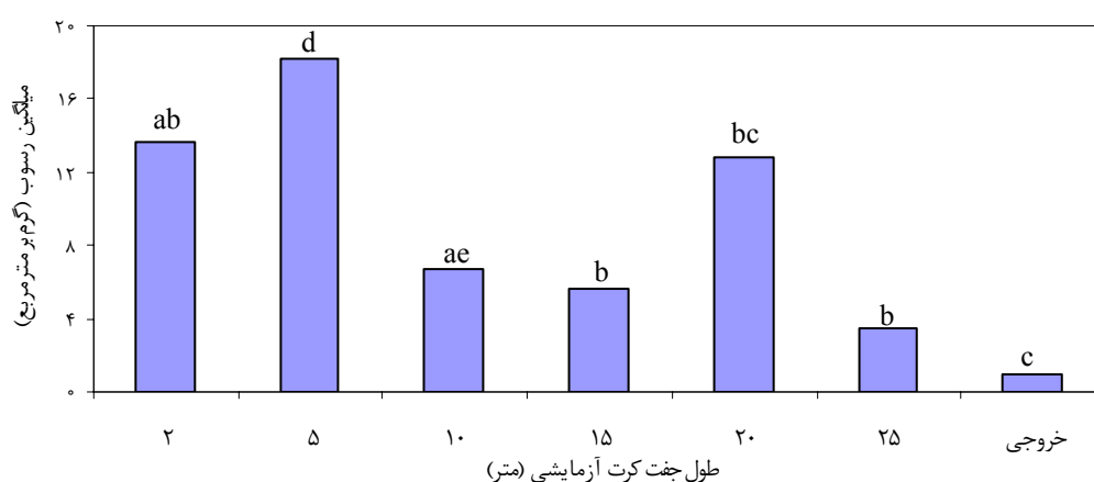
شکل ۳. گروه‌بندی داده‌های میانگین رسوب در واحد سطح (گرم در مترمربع) جفت کرت‌های آزمایشی با یکدیگر و با خروجی حوزه آبخیز با استفاده از آزمون Mann-Whitney U
