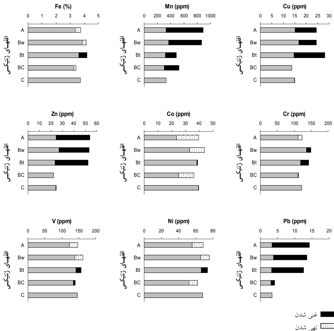
شکل ۱. غلظت کل اندازه‌گیری شده و محاسبه شده (لیتوزنیک) عناصر کیمیا در نیمرخ T02 (محاسبه شده با استفاده از رابطه ۱).
