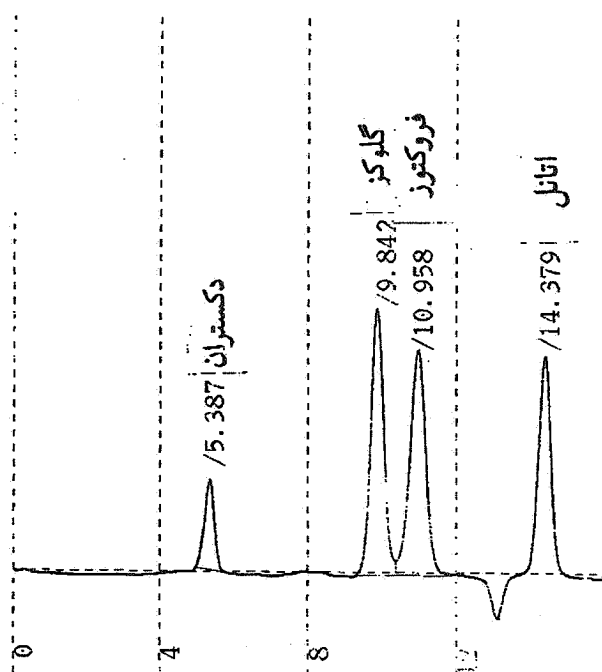
شکل ۲. کروماتوگرام واریته کبکاب بوشهر
