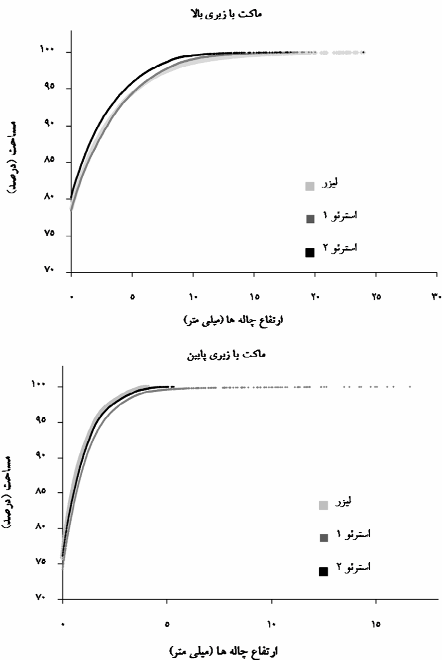
شکل ۱۳. نمودار تجمعی میزان مساحت سهم در ایجاد حداکثر نگهداشت سطحی با توجه به ارتفاعات چاله ها
