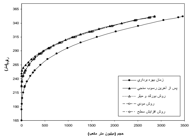
شکل ۷. منحنی‌های ارتفاع-حجم اولیه، ثانویه و پیش‌بینی شده برای سد دز
