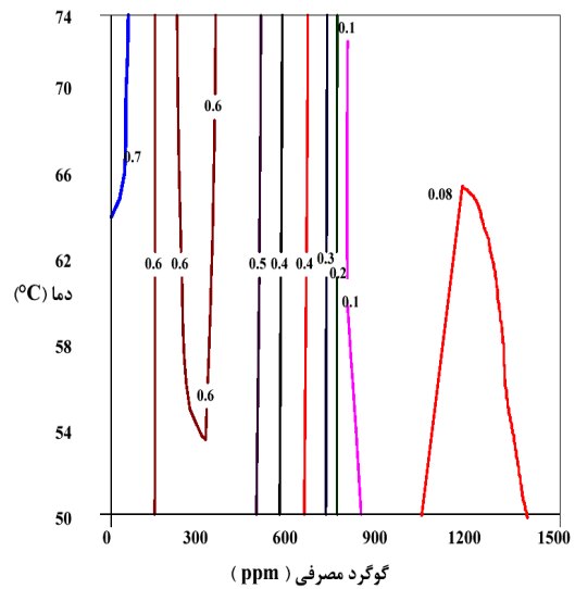
شکل ۳. خطوط هم تراز رنگ برای نمونه‌های تهیه شده به روش SBD (در مقادیر بالای مصرف گوگرد، انجام آنزیم‌بری پس از سولفیت‌زنی تأثیر زیادی در کاهش رنگ محصول ندارد).
