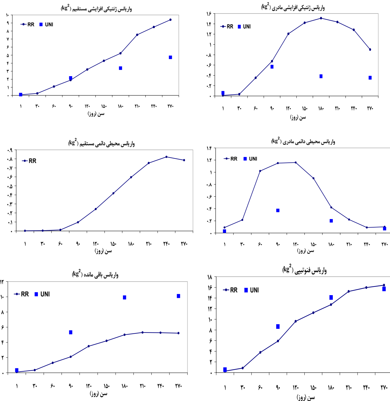
شکل ۱. اجزای واریانس برآورد شده از طریق مدل‌های RR (مدل ۴) و تک‌متغیره (UNI)
