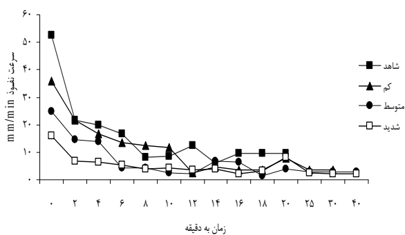
الف) سرعت نفوذ در شدت ترافیک‌های مختلف در مسیر چوبکشی ۵-۱ سال
