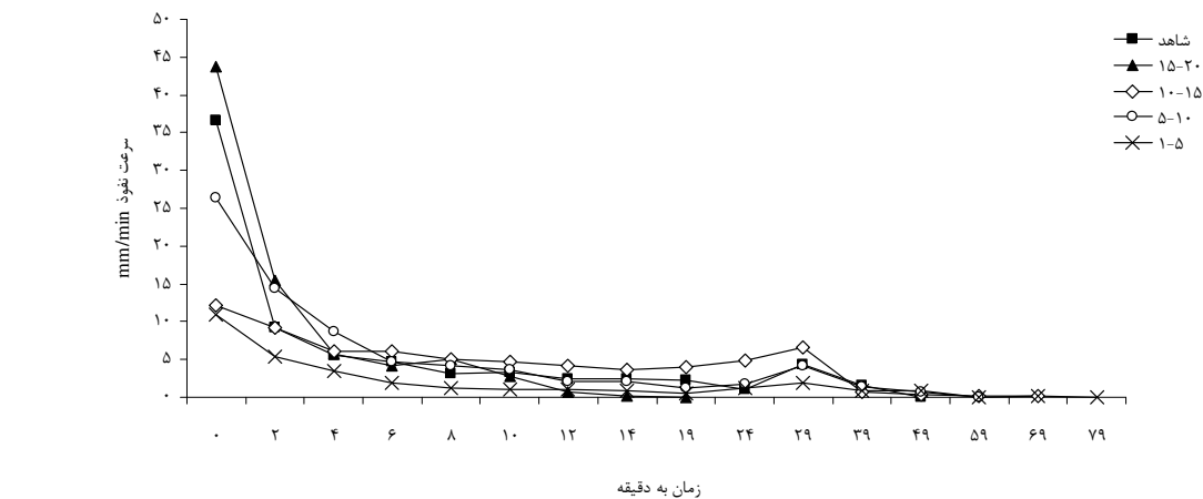
شکل ۲. مقایسه سرعت نفوذ در مسیرهای چوبکشی بیست سال پس از چوبکشی زمینی
