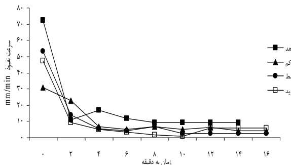
ب) سرعت نفوذ در شدت ترافیک‌های مختلف در مسیر چوبکشی ۵-۱۰ سال
