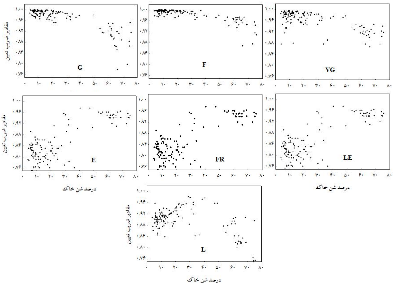
شکل ۸. رابطه بین ضرایب تعیین هفت مدل PSD ون گنوختن، فردلاند، گمپرتز، لگاریتمی- نمایی، فراکتال، نمایی و لگاریتمی با درصد شن نمونه‌های خاک. (VG = مدل ون گنوختن، F = مدل فردلاند، G = مدل گمپرتز، LE = مدل لگاریتمی- نمایی، FR = مدل فراکتال، E = مدل نمایی و L = مدل لگاریتمی)
