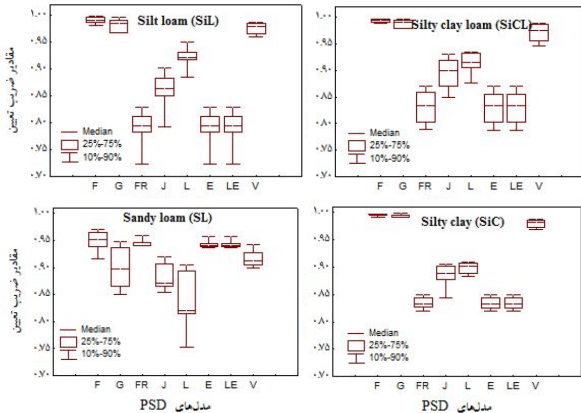
شکل ۴. نمودارهای جعبه‌ای ضرایب تعیین هشت مدل PSD مورد مطالعه در چهار کلاس بافت SiC، SiL، SiCL، SL و F (مدل = فردلاند، G = مدل گمپرتز، FR = مدل فراکتال، J = مدل جیکی، L = مدل لگاریتمی، E = مدل نمایی، LE = مدل لگاریتمی-نمایی و V = مدل ون گنوختن)
