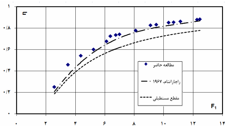
شکل ۴. تغییرات افت انرژی نسبتی بر حسب عدد فرود
