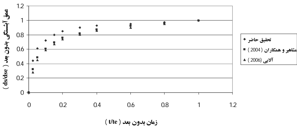
توسعه آبشستگی با طوق W=2D
