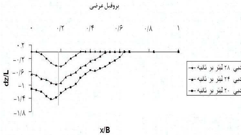
شکل ۵. پروفیل‌های طولی و عرضی حداکثر آبستگي در موقعیت ۱۶۰ درجه با دبی‌های مختلف
