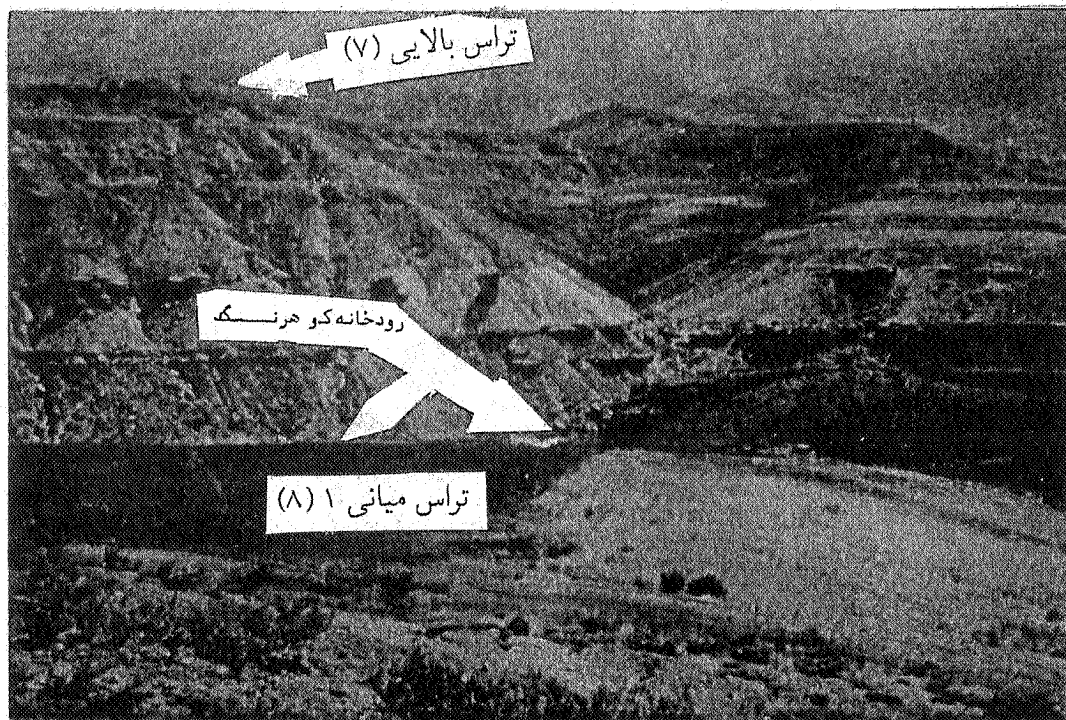
شکل ۳. نمایی از وضع زمین‌نمای تراس‌ها در اطراف رود کوه‌رنسگ (ناحیه اقلیمی چلگرد)
