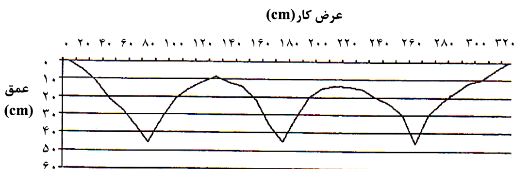
شکل ۵. سطح مقطع خاک به هم خورده توسط ریدرهای متصل به بولدوزر
