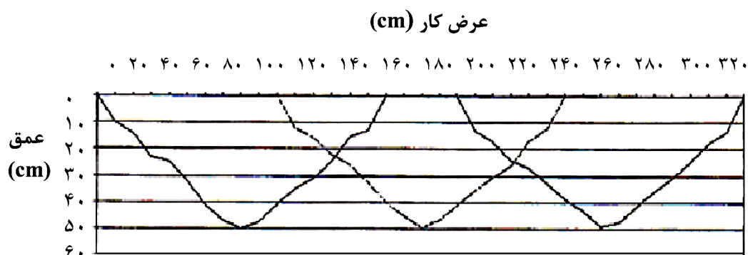
شکل ۴. متوسط سطح مقطع به هم خورده خاک دو سرریدف توسط تیمارهای زیر شکن کج ساق
