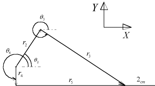
شکل ۵. نمایش برداری عضوهای مکانیزم
