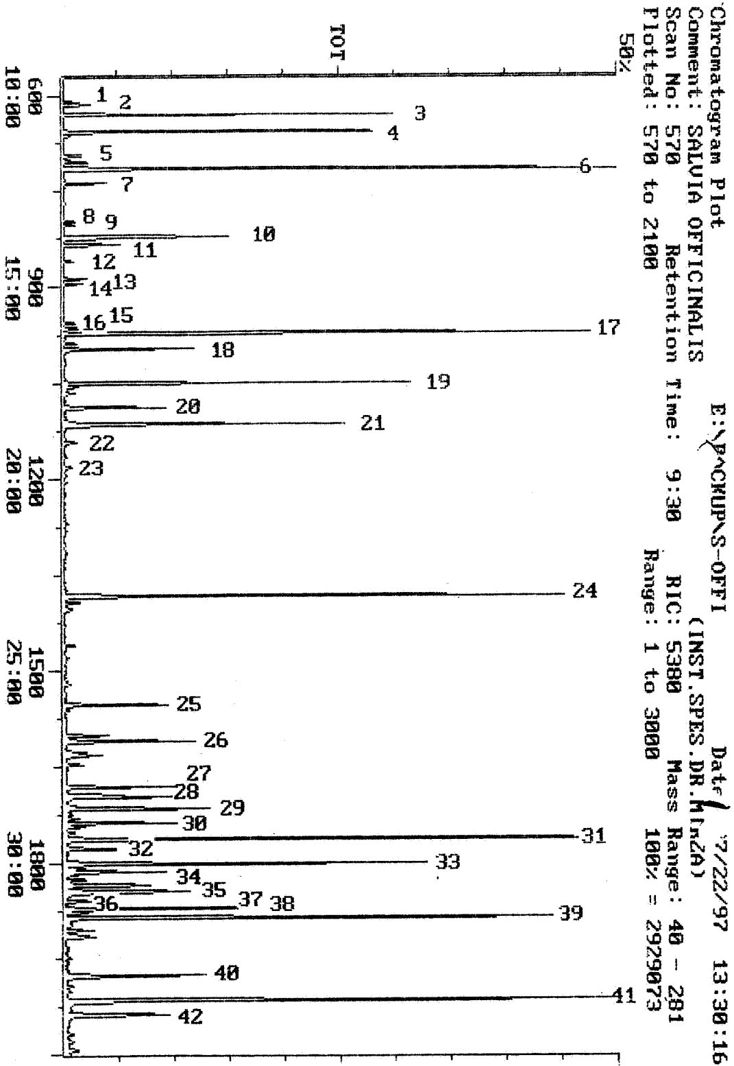
شکل ۱- کروماتوگرام اساسی سرشاخه گلدار گیاه مریم گلی دارویی Salvia officinalis L.
