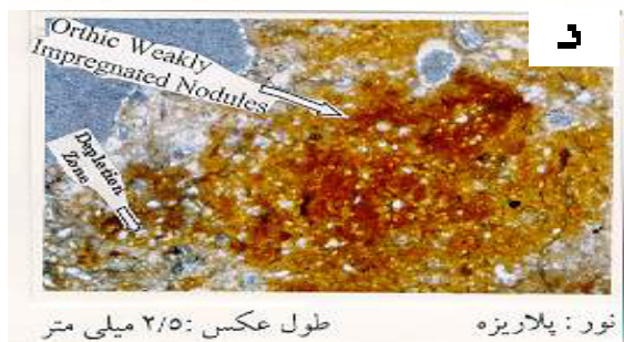
شکل ۴. (الف) سلول‌های گیاهی که به طور نسبی فیتولیتی شده‌اند در افق 3Ab (ب) پوشش کریستال‌های اسپارتیک آهک روی بقایای آلی در حفرات افق 3Ab (ج) پوشش آهکی در داخل خلل و فرج صفحه‌ای در افق 3Bkg2b (د) پدیده تخلیه و تجمع اکسیدهای آهن و منگنز به صورت ندول در افق 3Bkg2b نیم‌رخ سگری
