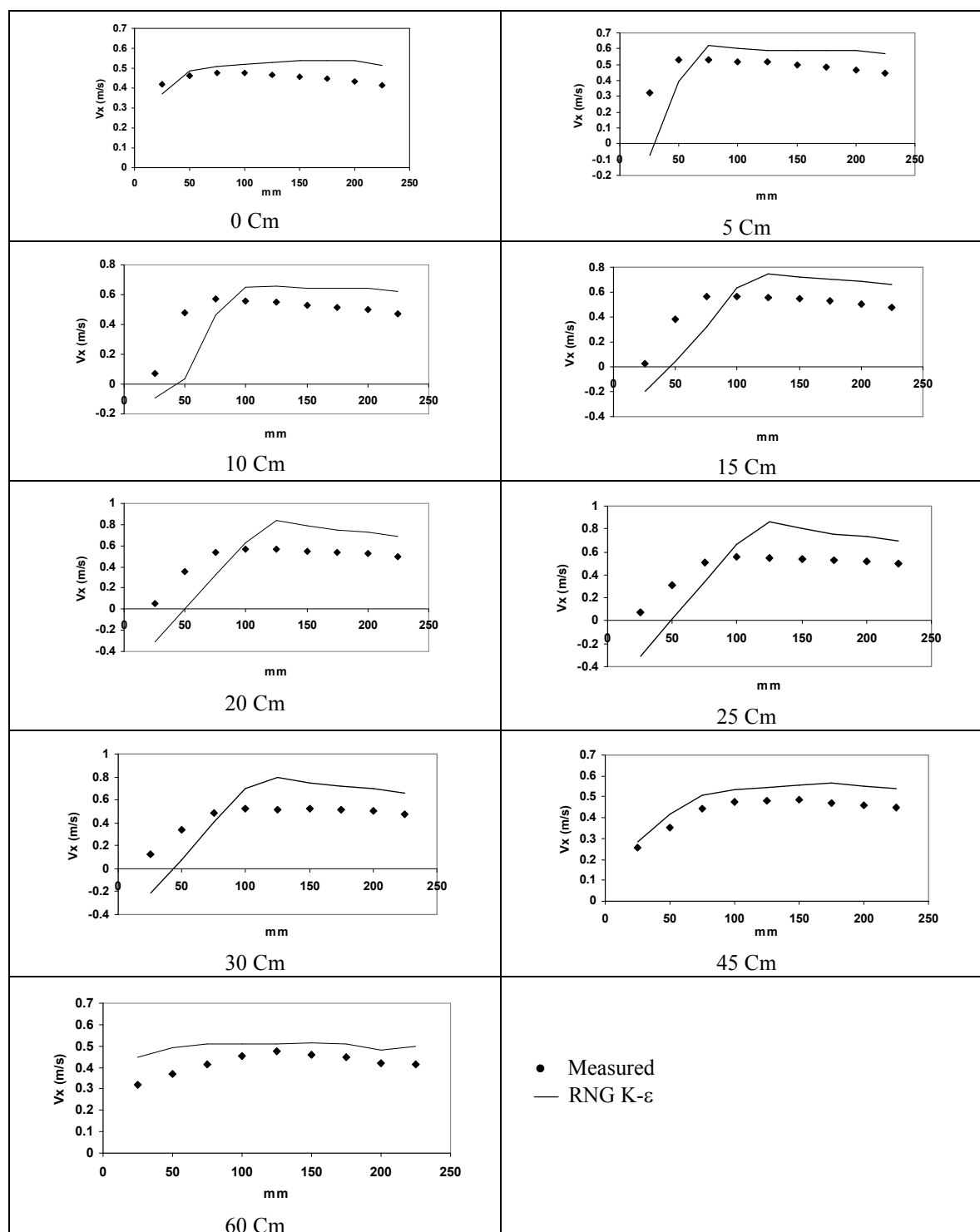
شکل ۸. مقایسه سرعت محاسبه شده در جهت جریان از مدل RNG K-ε با مقادیر اندازه‌گیری شده در کانال فرعی و در مقاطع مختلف از ورودی برای عمق ۲۰ سانتی‌متر
