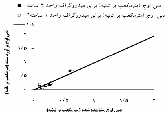
شکل ۳. الف) زمان تا اوج مشاهده‌ای و برآوردی هیدروگراف واحد ۱ و ۲ ساعته حوضه و زیرحوضه‌های آبخیز مارنج ب) زمان پایه مشاهده‌ای و برآوردی هیدروگراف واحد ۱ و ۲ ساعته حوضه و زیرحوضه‌های آبخیز مارنج ج) دبی اوج مشاهده‌ای و برآوردی هیدروگراف واحد ۱ و ۲ ساعته حوضه و زیرحوضه‌های آبخیز مارنج
