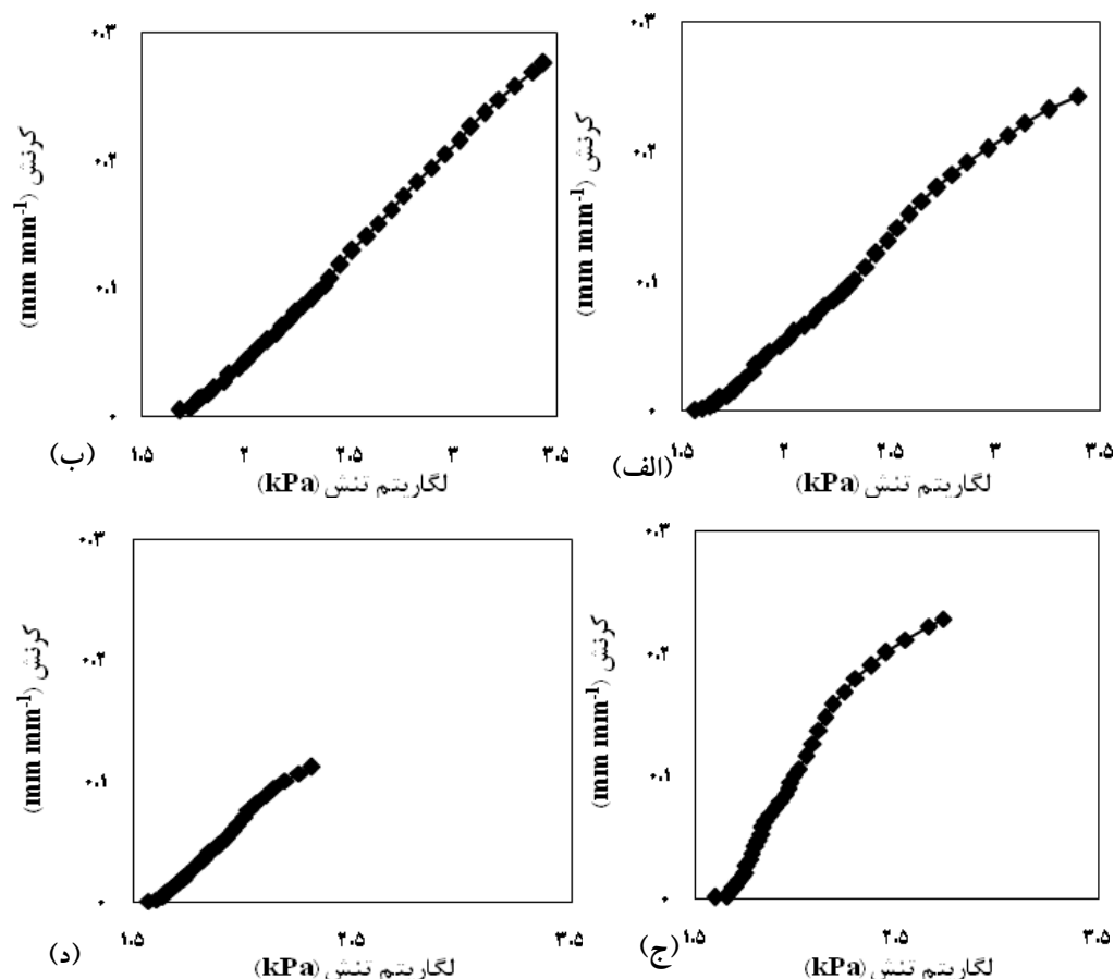
شکل ۳. نمونه‌هایی از نمودار لگاریتم تنش-نشست خاک رس سیلتی در آزمایش فشردگی محصور (CCT)، بدون بار متراکم‌کننده، (الف) رطوبت 0/9 PPL بدون تروخشک شدن، (ب) رطوبت 0/9 PPL با تروخشک شدن، (ج) رطوبت 1/1 PPL بدون تروخشک شدن و (د) رطوبت 1/1 PPL با تروخشک شدن.
