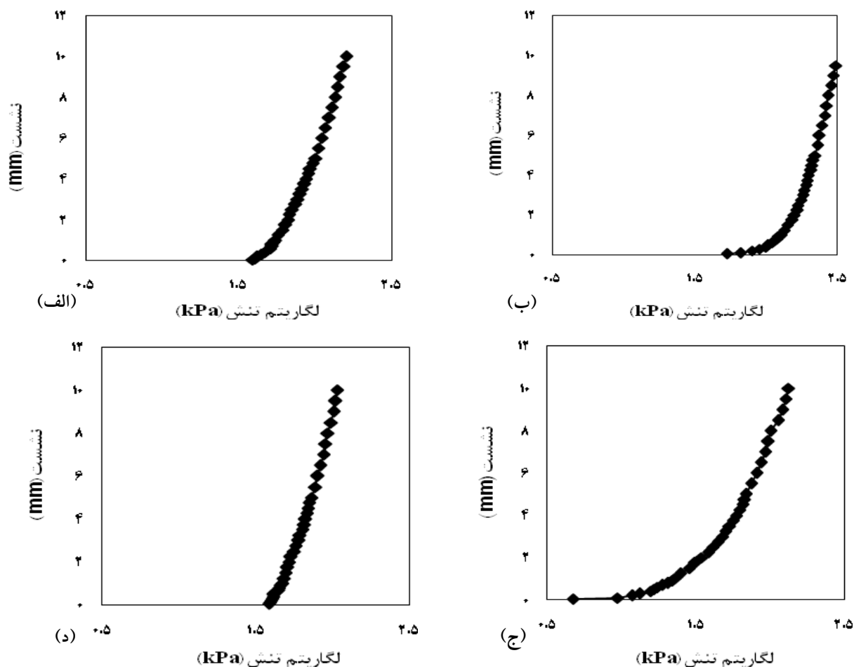
شکل ۲. نمونه‌هایی از نمودار لگاریتم تنش-نشست خاک رس سیلتی در آزمایش نشست صفحه‌ای (PST) بدون بار متراکم‌کننده، الف) رطوبت ۰/۹ P L بدون تروخشک شدن، ب) رطوبت ۰/۹ P L با تروخشک شدن، ج) رطوبت ۱/۱۰ P L بدون تروخشک شدن و د) رطوبت ۱/۱۰ P L با تروخشک شدن.
