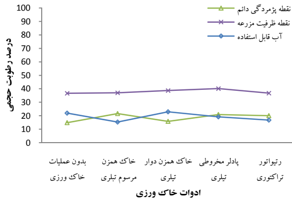
شکل ۹. روند درصد رطوبت حجمی خاک در نقطه ظرفیت زراعی و پژمردگی دائم و آب قابل استفاده ادوات مختلف خاک‌ورزی
