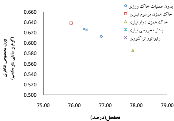
شکل ۱۴. مقایسه روند تخلخل و وزن مخصوص ظاهری برای ادوات مختلف خاک‌ورزی با دفعات مختلف پادلینگ
