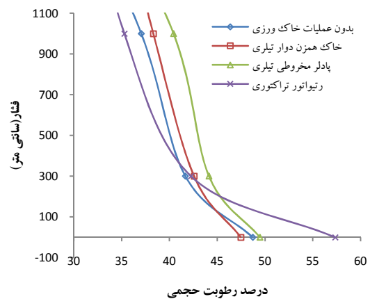
شکل ۱۳. مقایسه منحنی مشخصه خاک بدون عملیات خاک‌ورزی و خاک پادل شده با ادوات خاک‌ورزی مختلف در فشار اشباع، ظرفیت زراعی (۳۰۰ سانتی متر)، آستانه ترک بحرانی (۱۰۰۰ سانتی متر)
