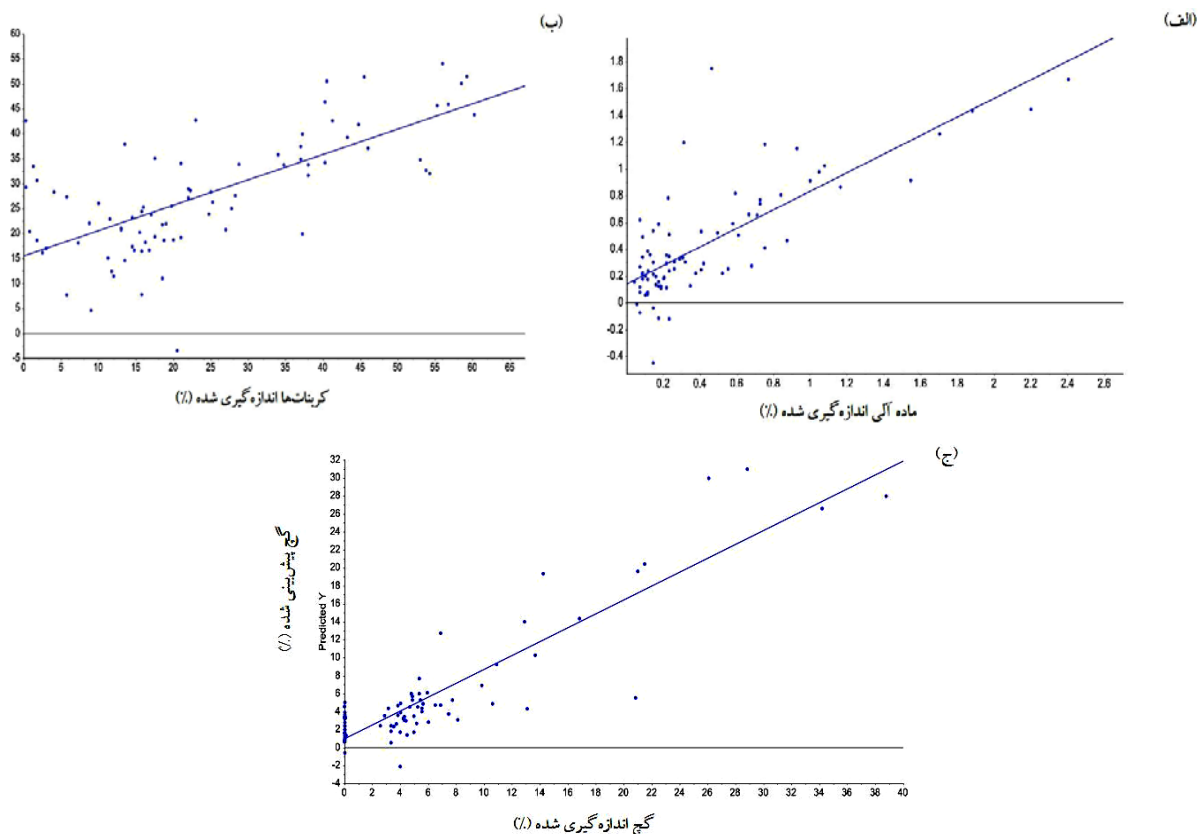
شکل ۴. مقادیر اندازه‌گیری شده در مقابل مقادیر پیش‌بینی شده ماده آلی (الف) ، کربنات‌ها (ب) و کچ (ج) توسط مدل PLSR در گروه اعتبارسنجی
