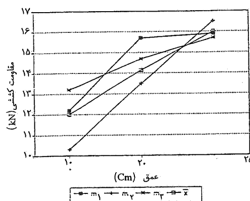
شکل ۲- تغییرات میانگین مقاومت کششی در اعماق مختلف عمق شخم در هر یک از سطوح رطوبت خاک
