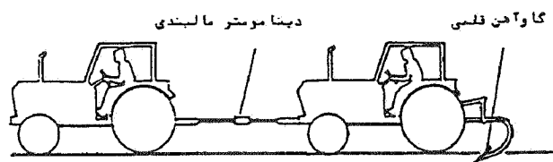
شکل ۱- اندازه گیری مقاومت کششی گاواهن قلمی سوار شونده با استفاده از روش دو تراکتوری و دینامومتر مالبندی
