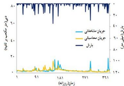
شکل ۴. دبی روزانه مشاهده‌ای و شبیه‌سازی شده مدل
