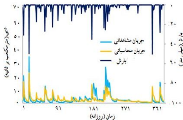
شکل ۵. دبی روزانه مشاهده‌ای و شبیه‌سازی شده مدل
