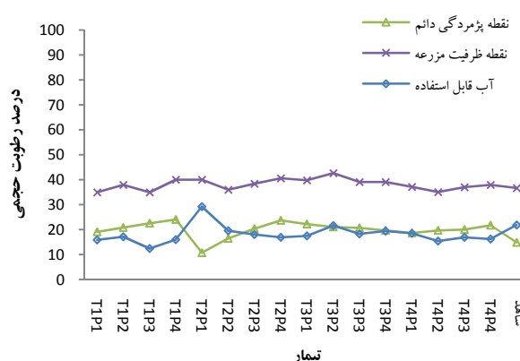
شکل ۸. روند درصد رطوبت حجمی خاک در نقطه ظرفیت زراعی و پژمردگی دائم و آب قابل استفاده ادوات مختلف خاک‌ورزی با پادلینگ مختلف
