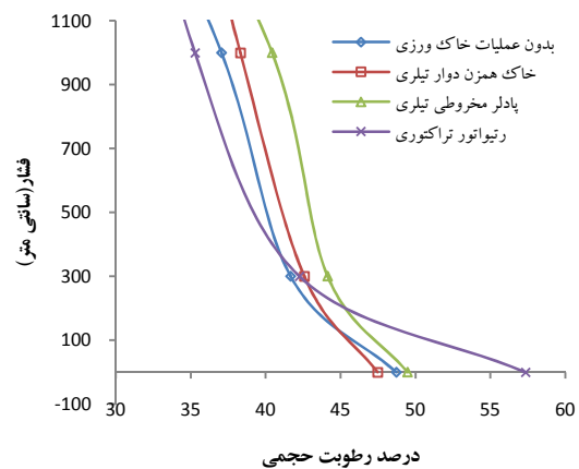
شکل ۱۳. مقایسه منحنی مشخصه خاک بدون عملیات خاک‌ورزی و خاک پادلر شده با ادوات خاک‌ورزی مختلف در فشار اشباع، ظرفیت زراعی (۳۰۰ سانتی متر)، آستانه ترک بحرانی (۱۰۰۰ سانتی متر)
