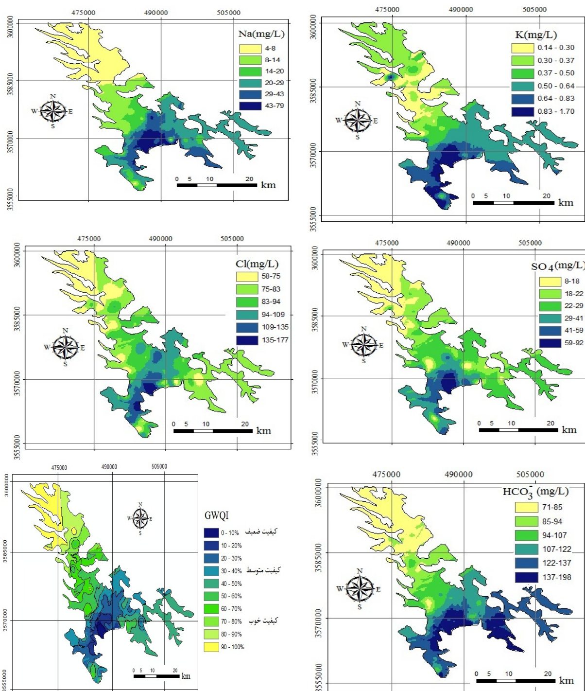
شکل ۳. نقشه‌های \text{Na}^+ , \text{K}^+ , \text{Cl}^- و \text{HCO}_3^- و \text{SO}_4^{2-} در آب زیرزمینی شهرکرد
