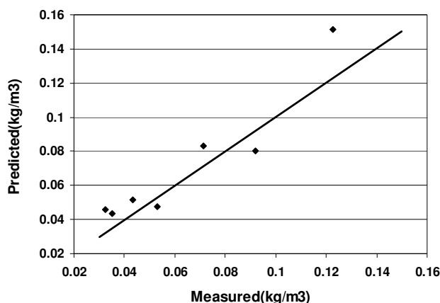
شکل ۱۰. مقایسه همبستگی بین نتایج مدل و مقادیر اندازه‌گیری شده در مرحله واسنجی مدل
