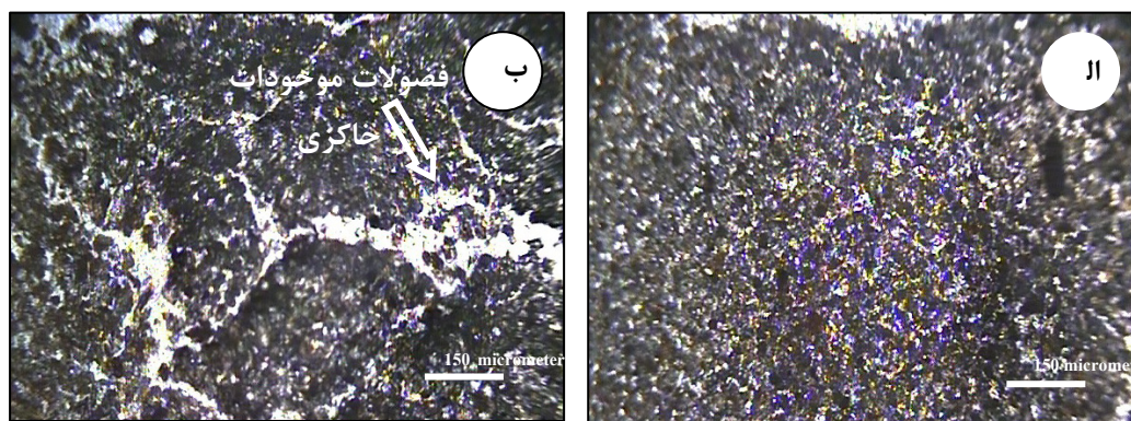
شکل ۵. تصاویر میکروسکوپی از ساختمان و حفرات خاک بدون پوشش (الف) و با پوشش گلسنگ (ب) (شکل الف ساختمان متراکم را نشان می دهد در حالی که در شکل ب ساختمان بلوکی با جداشدگی خوب دیده می شود)
