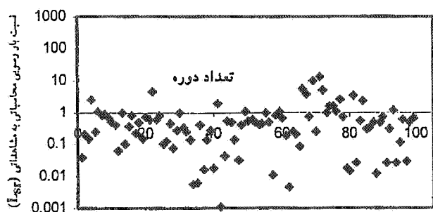
نمودار ۲-۱۱. روش بگ اصلاح شده، رودخانه کرخه
