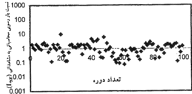
نمودار ۳-۷. روش انگلاند و هانسن، رودخانه کارون
