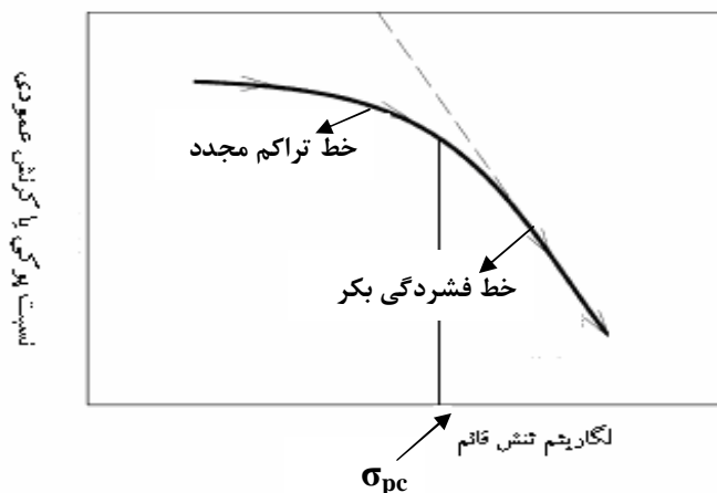
شکل ۱. ویژگی‌های منحنی مشخصه فشردگی خاک (رابطه نسبت پوی (e) یا کرنش عمودی (ε) خاک با تنش فشاری. \sigma_{pc} تنش پیش‌تراکمی است (۹).
