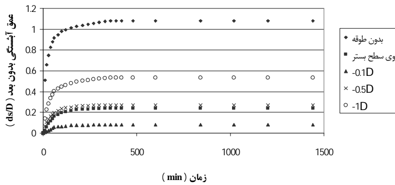
شکل ۷. تاثیر ارتفاع نصب طوقه نسبت به تراز بستر در مقایسه با پایه بدون طوقه در قطرهای مختلف روی آبستگي
