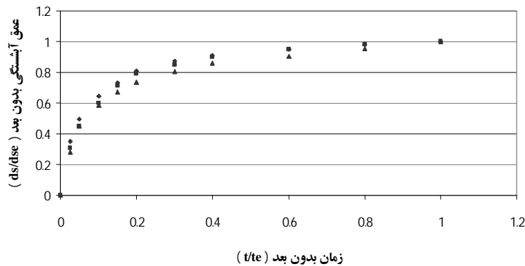
توسعه آبستگي با طوق W=2D
