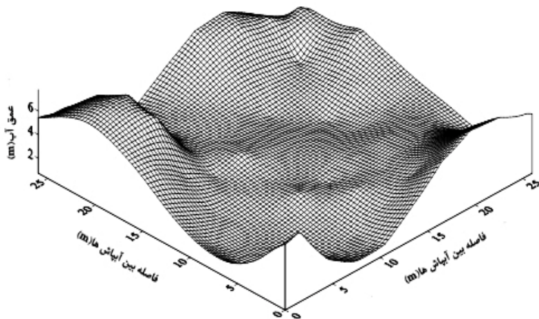
شکل ۳. الگوی توزیع آب پس از همپوشانی آبیاش‌های مورد آزمایش در مزرعه SN
