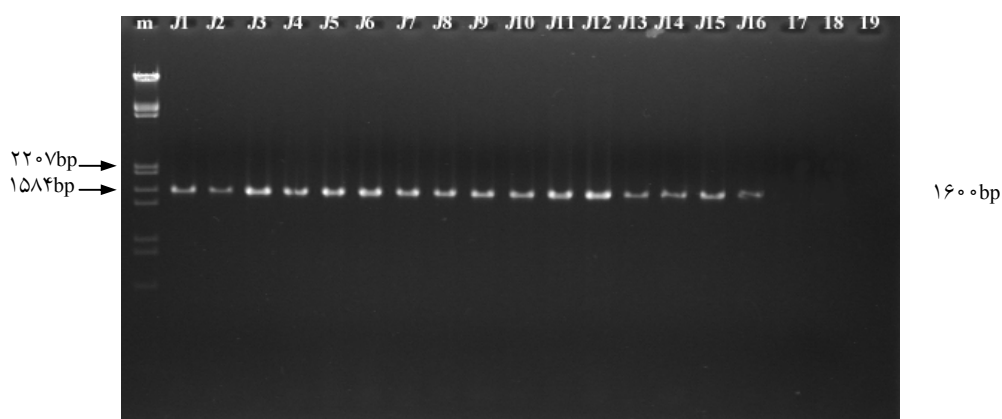
شکل ۵. تکثیر باند ۱۶۰۰ جفت بازی توسط جفت آغازگر Mjavf / Mjavr در جمعیت‌های مختلف گونه M. javanica (J1- J16)
