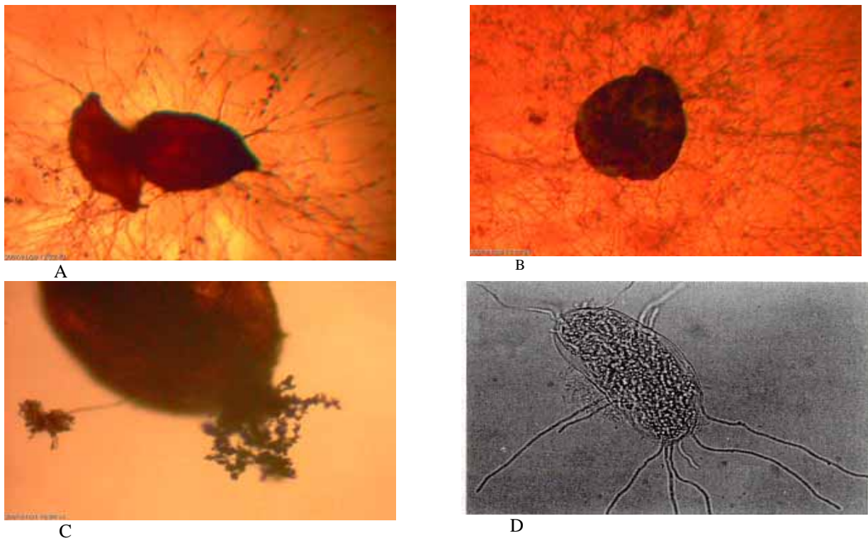
شکل ۲. سیست‌ها و تخم Heterodera schachtii پارازیت شده به وسیله Trichoderma harzianum A، B- بزرگنمایی ۲۰۰ ، C- بزرگنمایی ۴۰۰ ، D- بزرگنمایی ۱۰۰۰ .
