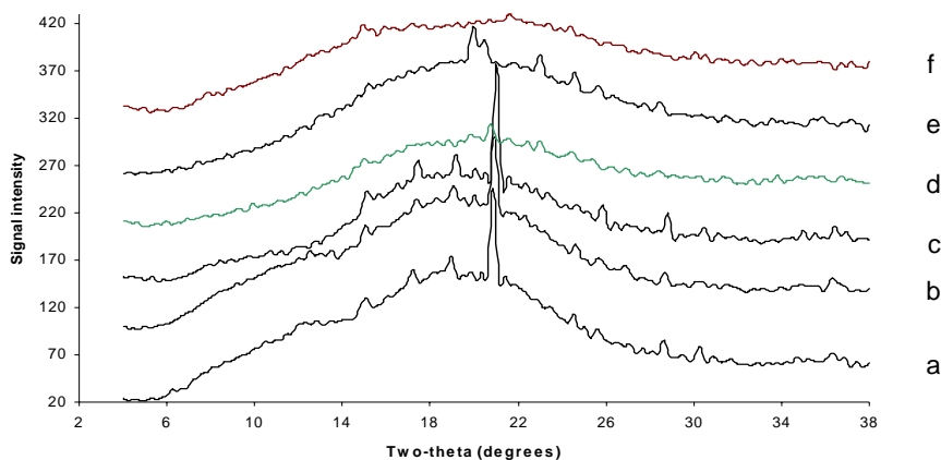
نمودار ۴. الگوی دیفرکسیون X-ray نمونه‌های انجیر تیمار یافته با ۰/۴٪ گلوکز سیراپ به تعادل رسیده در فعالیت آبی‌های (f: ۰/۸۴۳، e: ۰/۷۴۳، d: ۰/۶۴۳، c: ۰/۳۸۲، b: ۰/۲۲۷، a: ۰/۱۱۲) در دمای ۲۵ °C
